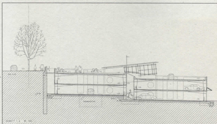
Schnitt 1.4; Ausführungsplanung
