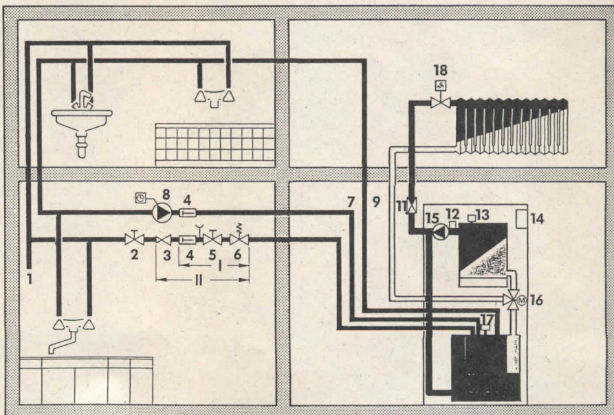
Installationsbeispiel
